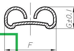
CORTE P-P
